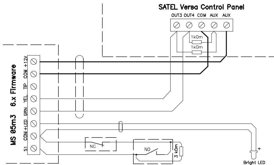
Рисунок 4. Подключение к охранным панелям SATEL Versa. MS05m3 Firmware 6.x.
