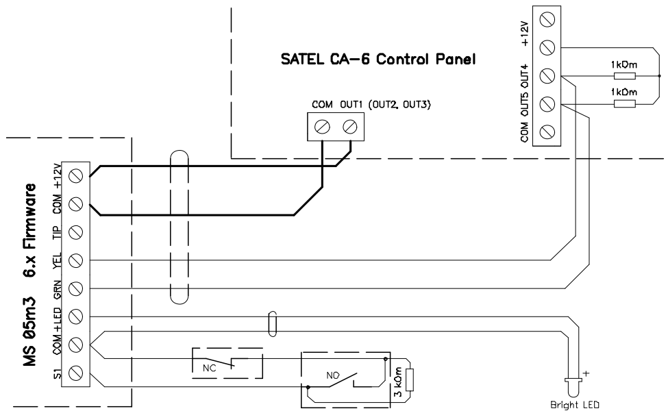
Рисунок 2. Подключение к охранным панелям SATEL CA-6. MS05m3 Firmware 6.x.
