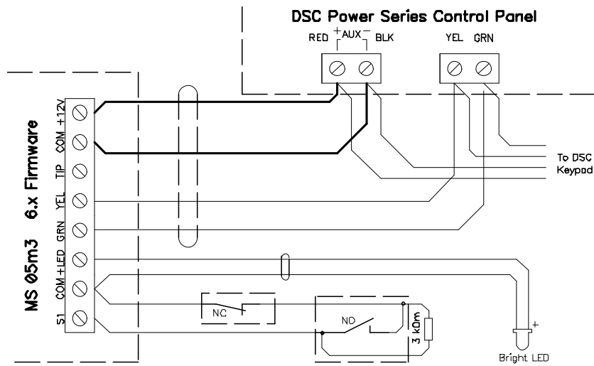
Рисунок 1. Подключение к охранным панелям DSC. MS05m3 Firmware 6.x.
