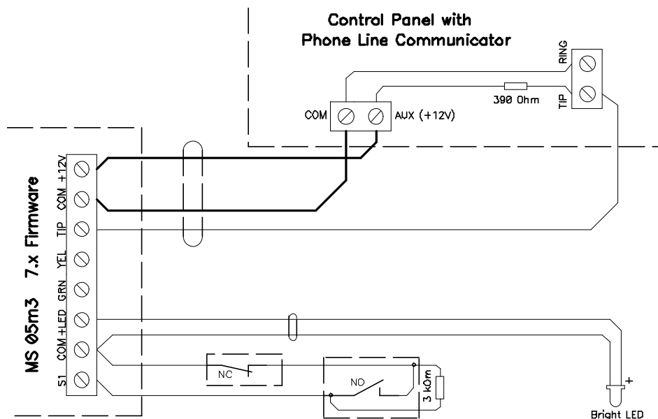
Рисунок 6. Подключение к охранным панелям со встроенным телефонным коммуникатором. MS05m3 Firmware 7.x.
