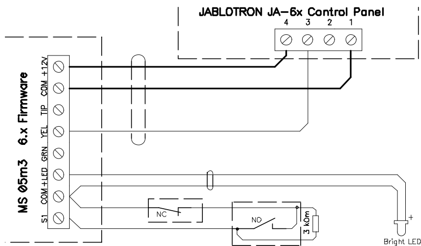
Рисунок 5. Подключение к охранным панелям JABLOTRON JA-6x. MS05m3 Firmware 6.x.
