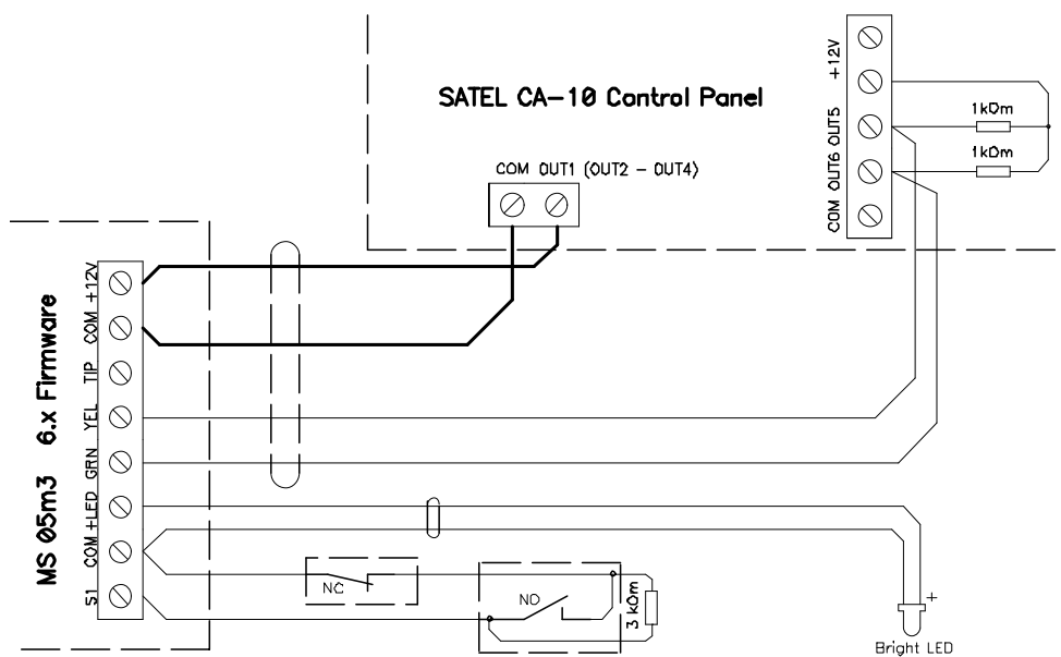
Рисунок 3. Подключение к охранным панелям SATEL CA-10. MS05m3 Firmware 6.x.
